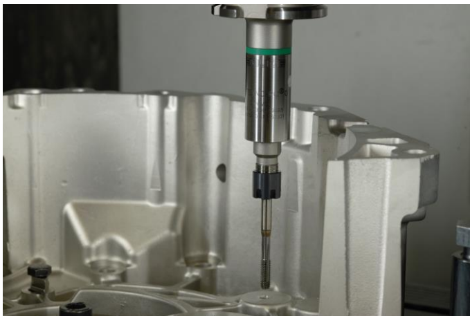
Bild 2: Die Spannzangen-Aufnahme Softsynchro® Slim mit sehr schlankem Schaft gibt es auch für innere Kühlmittelzufuhr oder Minimalmengenschmierung.
